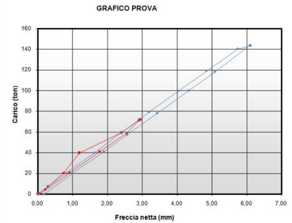
Grafico carichi/frecce
